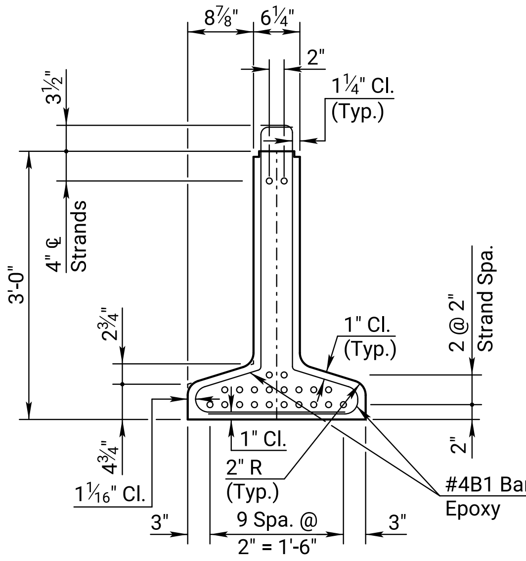
SECTION A-A
