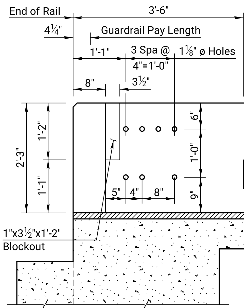
ELEVATION
