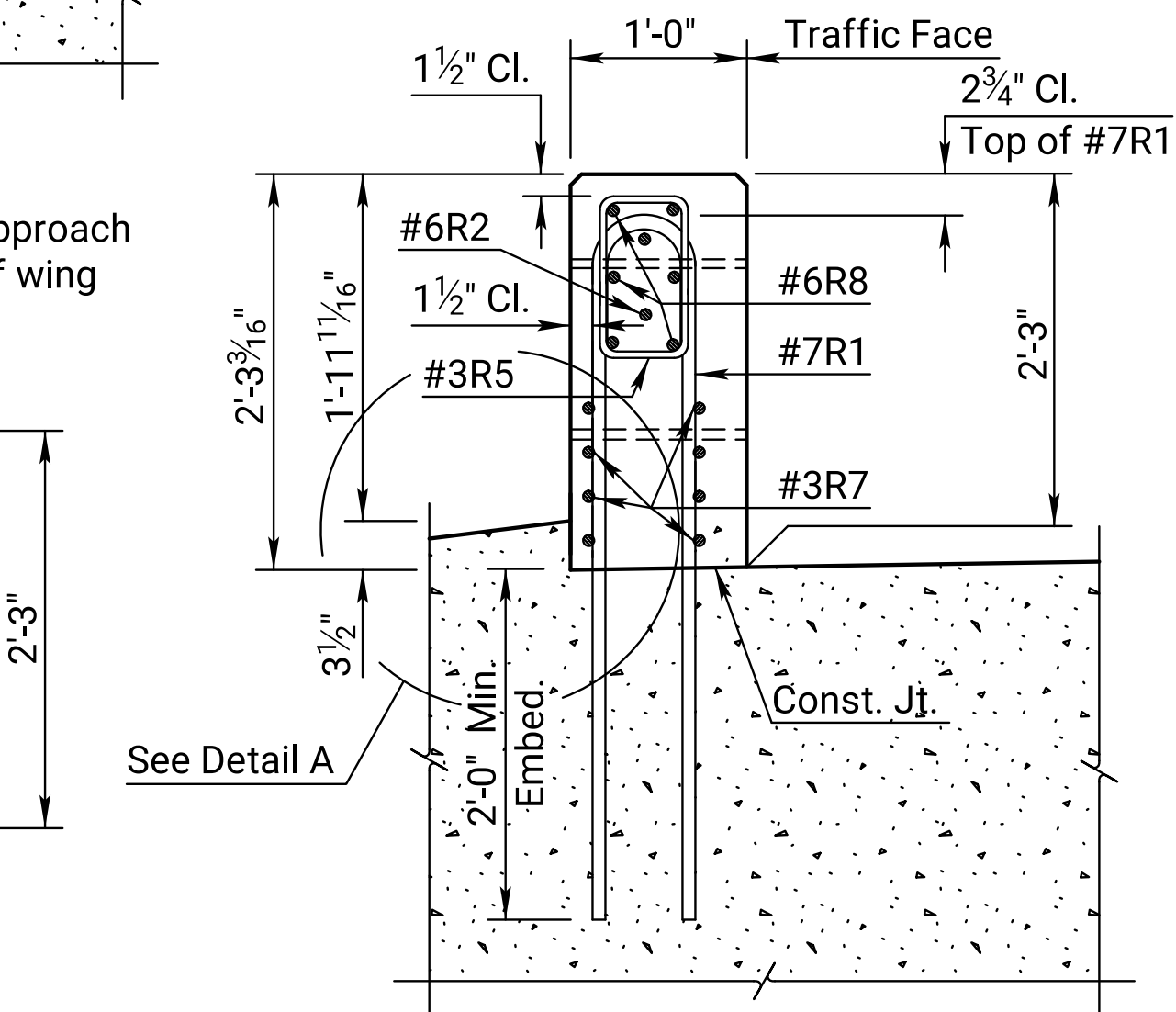
SECTION A-A
