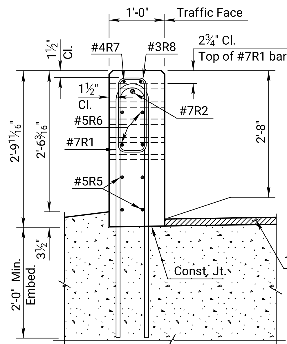
SECTION A-A
