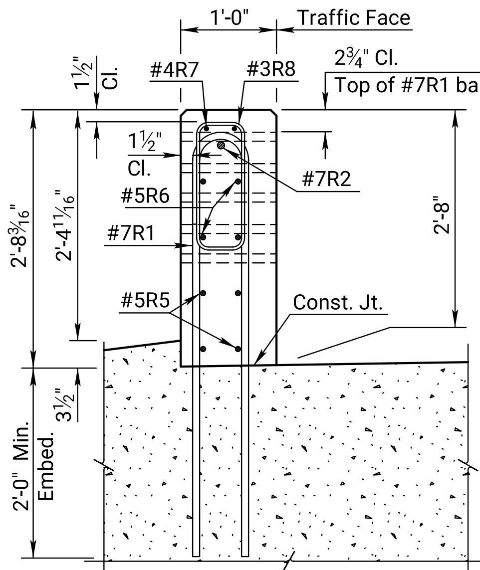
SECTION A-A
