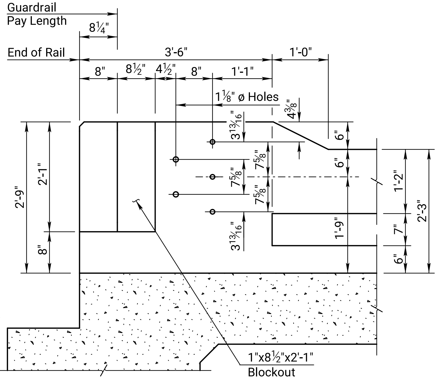
ELEVATION
